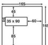
Vindu nr. 11. 165 x 165 høyt vindu venstre
