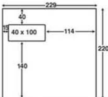
Vindu nr. 21. 220 x 229 høyt vindu venstre
