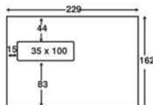
Vindu nr. 16. C5 høyt vindu venstre
